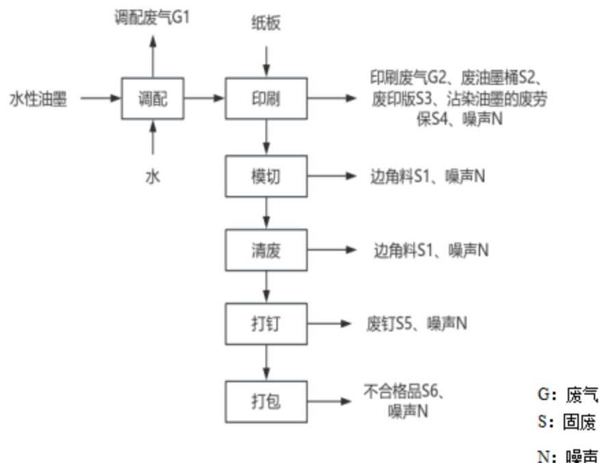
图 2-2 工艺流程图
